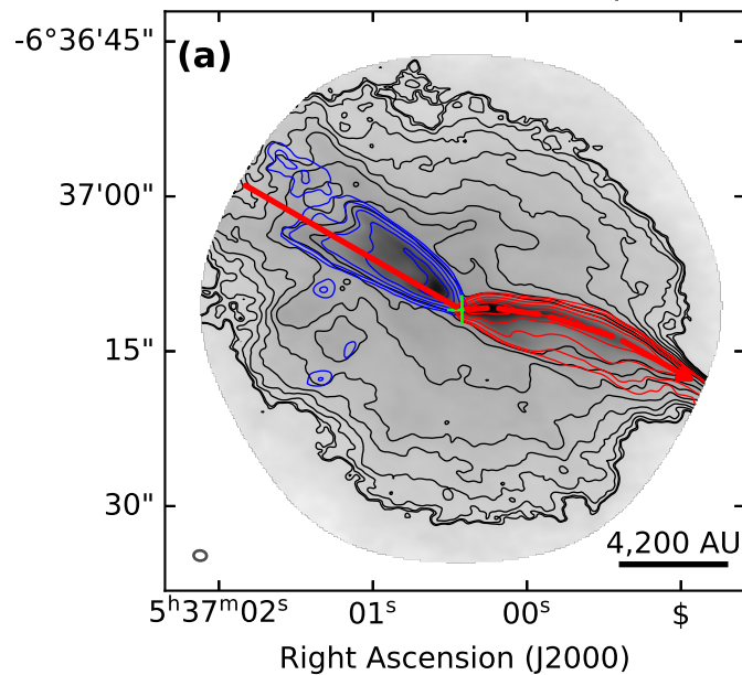
^{12}\text{CO} Moment 0 Map
