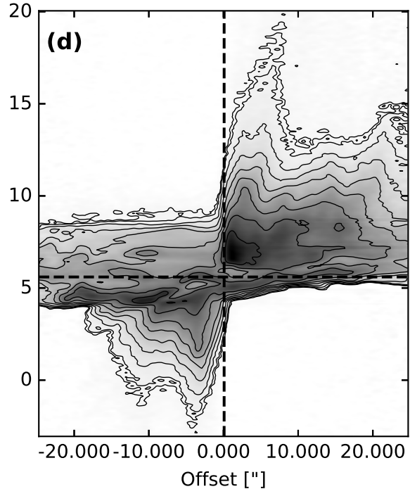
^{12}\text{CO}
