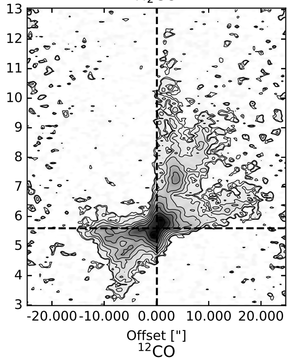
\text{H}_2\text{CO}
