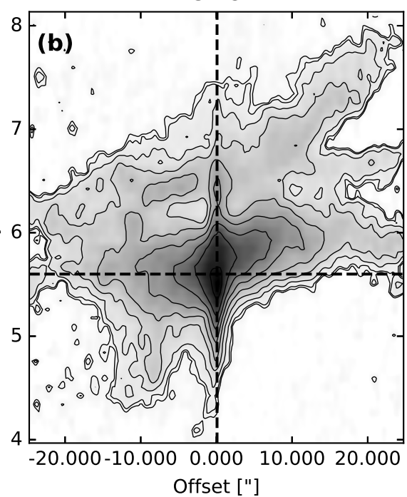
\text{C}^{18}\text{O}
