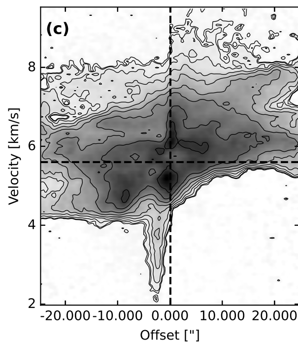
^{13}\text{CO}
